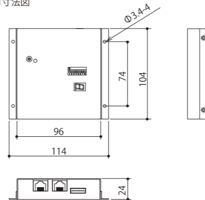
■寸法図
