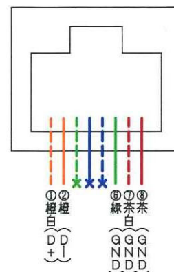
OUT1~8 ピンアサイン
